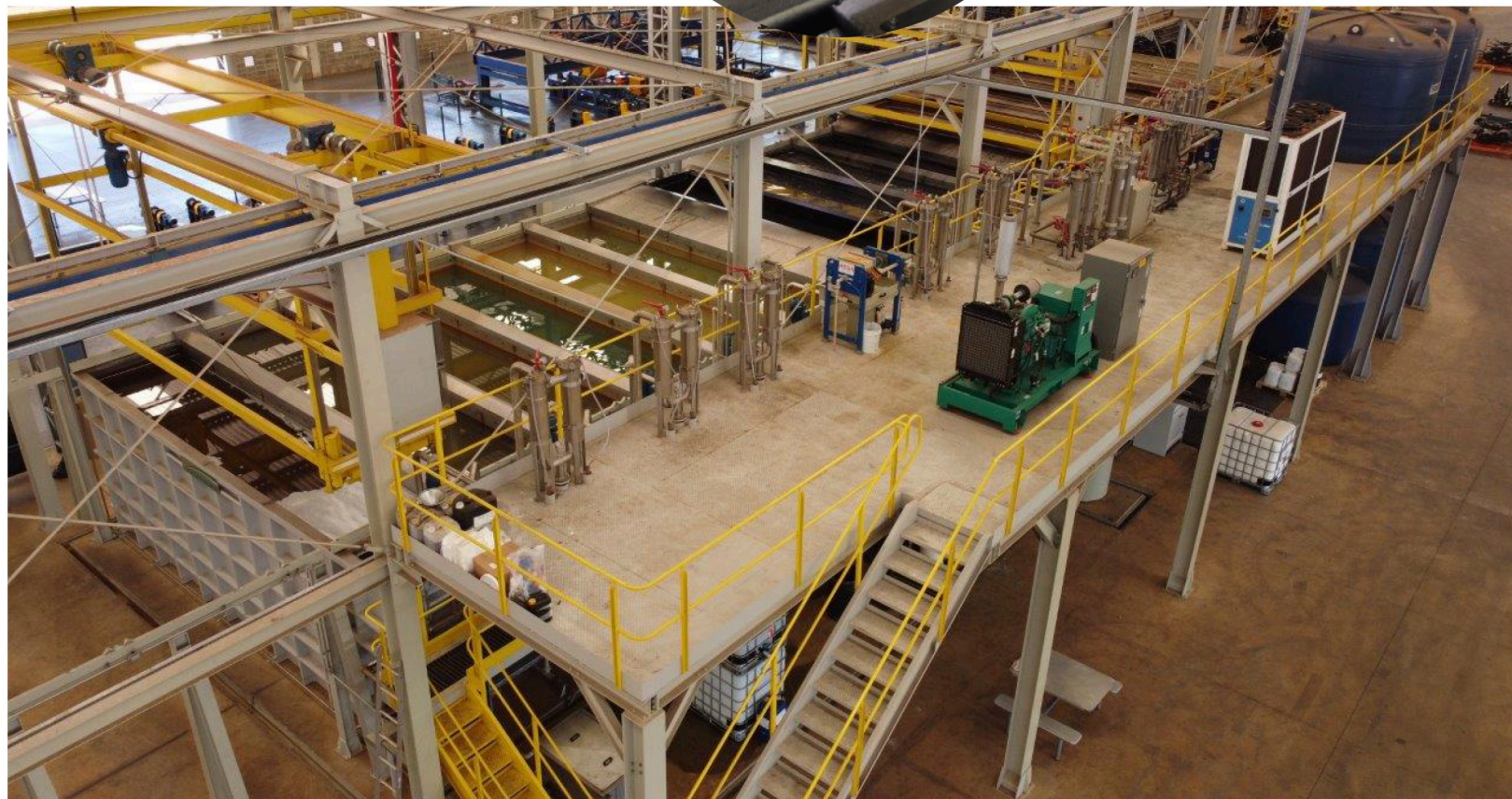
LINHA DE PRODUÇÃO DE PINTURA SUBMERSA
